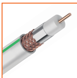
■ КАБЕЛЬ РАДИОЧАСТОТНЫЙ SAT в бухтах по 100 м
