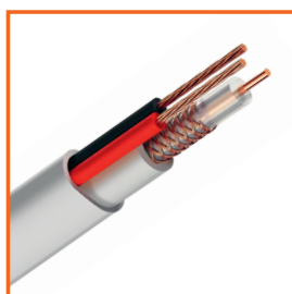
■ КАБЕЛИ ДЛЯ ВИДЕОНАБЛЮДЕНИЯ КВК, 200 м
